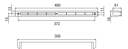
AEA 1152 (kiegészítő toldó) egyaránt választható AEA 1150 és AEA 1151 típusokhoz
