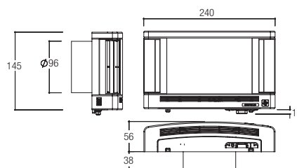
EHT 780, 957, 022 és EFT 840, 026 típusok
