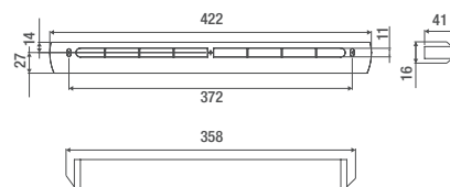
AEA 1150 / AEA 1151 azonos elemrész (esővédő oldal)
